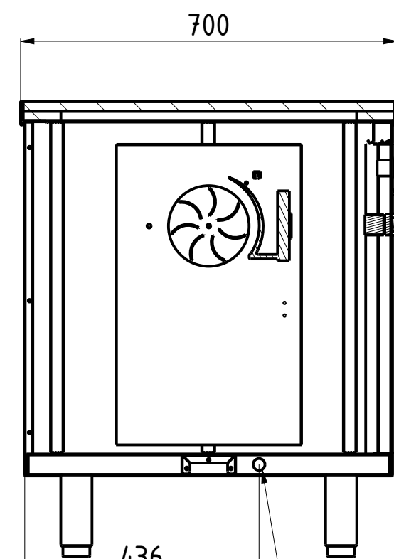
USCITA MODULO CALDO POWER SUPPLY OUTPUT
